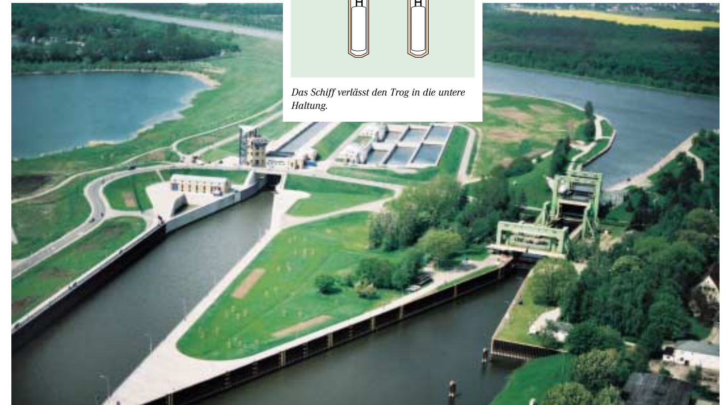
Schiffshebewerk und Sparschleuse Rothensee, Mai 2002
