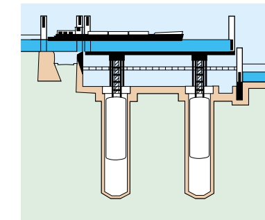
Aus der oberen Haltung fährt ein Schiff in den Trog des Hebewerkes Rothensee.
