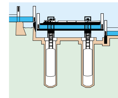
Der Trog wird durch Drehen der 4 Spindelmuttern heruntergeschraubt. Er hat im Bild eine mittlere Stellung erreicht.
