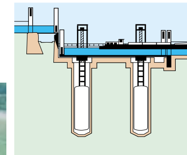
Das Schiff verlässt den Trog in die untere Haltung.
