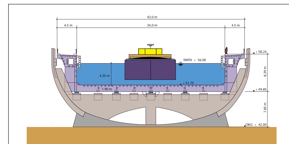
Brückenquerschnitt im Vorlandbereich
