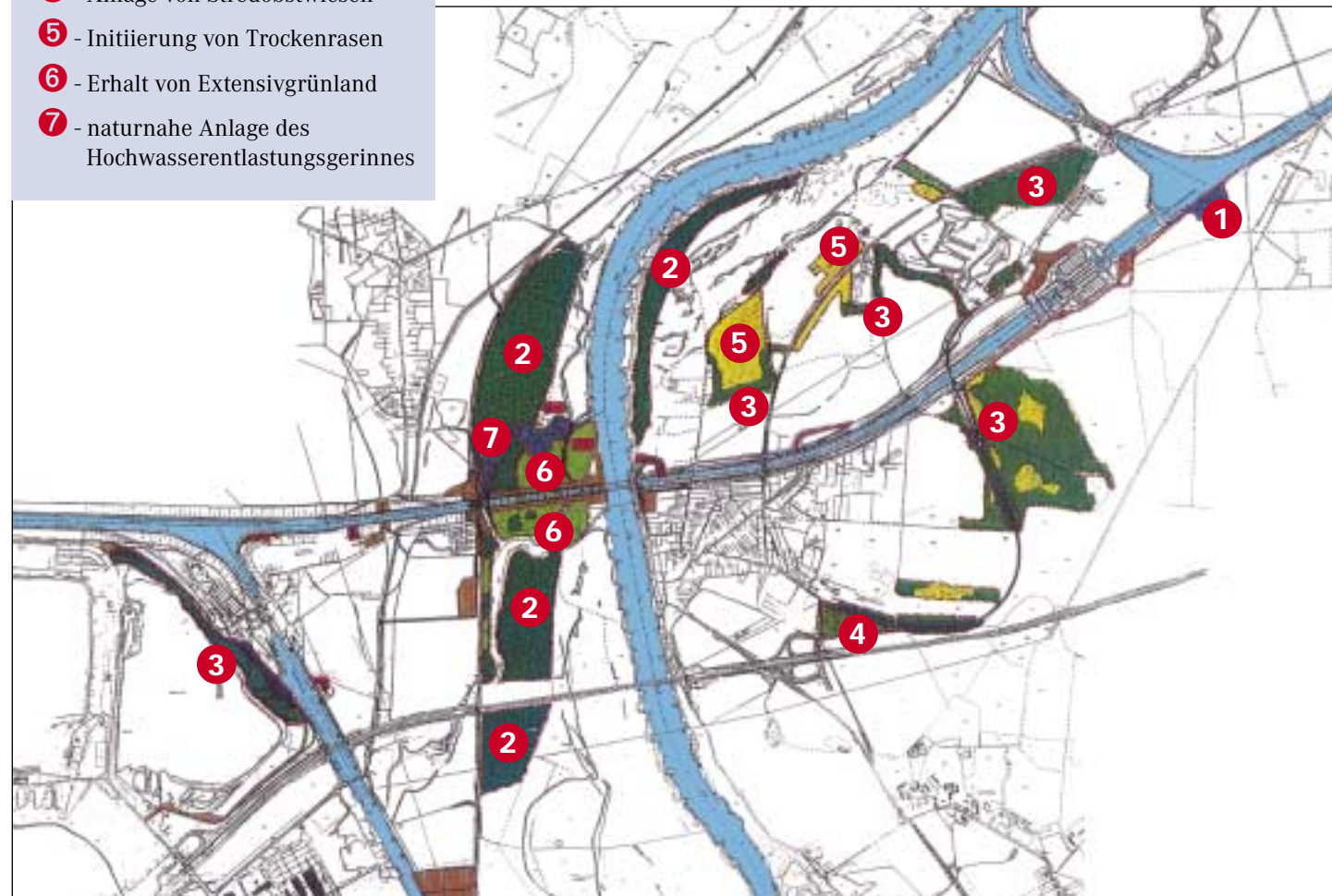
16 Ausgleichs- und Ersatzmaßnahmen am Wasserstraßenkreuz Magdeburg, Übersichtsplan
