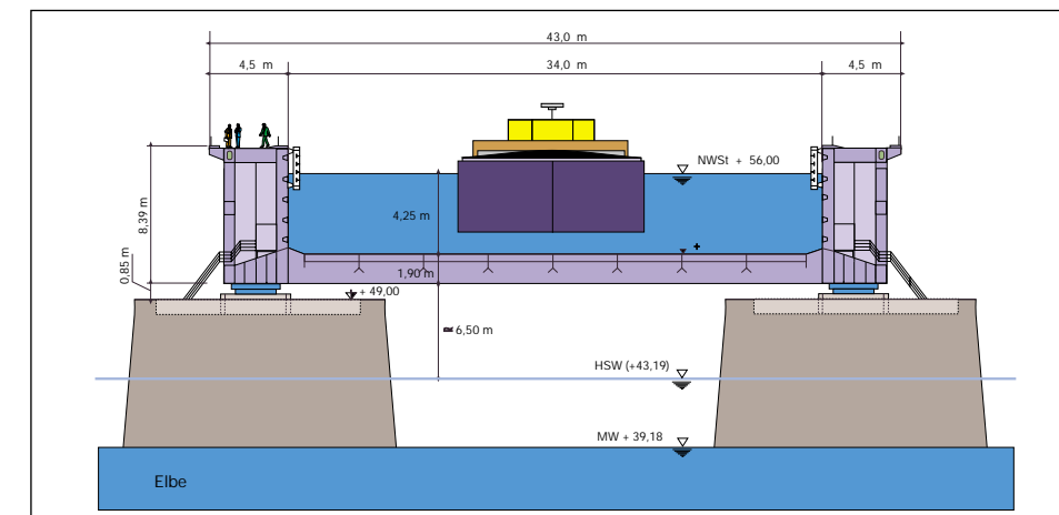
Brückenquerschnitt im Strombereich
