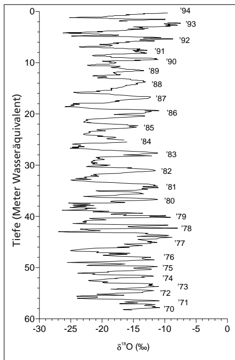
Figur 5 Datierung der oberen 60 m des Grenzgletscher-Eisbohrkerns durch Abzählen der Jahresschichten, wobei man die Tatsache nutzt, dass sich die Schneekristalle von Sommer- und Winterniederschlägen in ihrer Zusammensetzung geringfügig unterscheiden.
