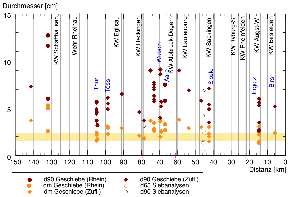
Bild 6.1 Charakteristische Korndurchmesser der vorhandenen Geschiebeproben aus dem Rhein und den Zuflüssen (Zufl.). Gelber Balken: Bandbreite des massgebenden Korndurchmessers des Thurgeschiebes.
