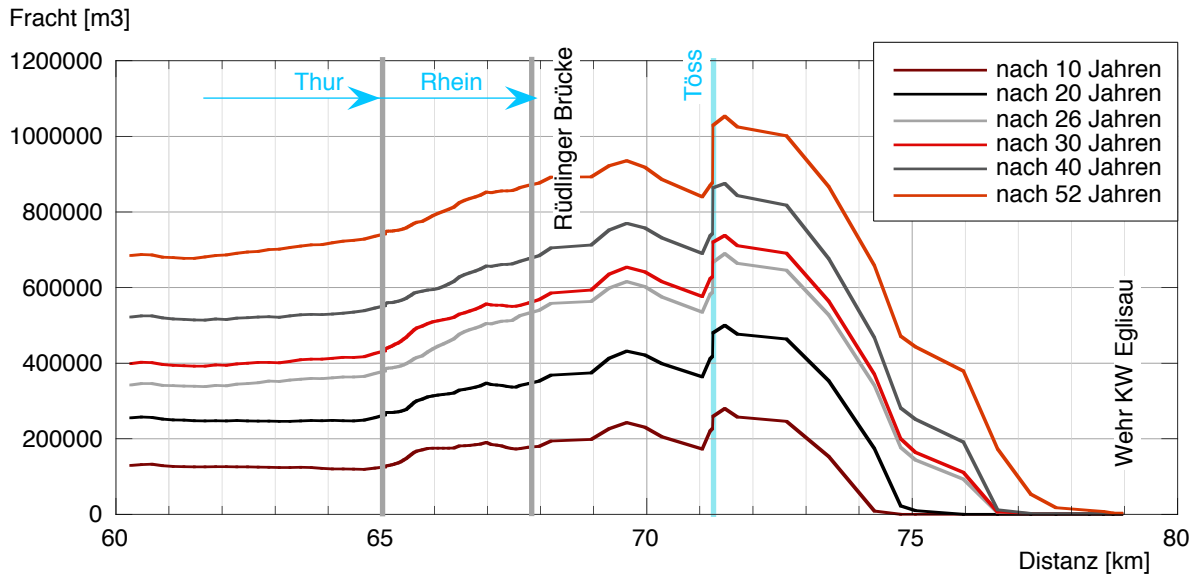
Bild 3.2 Längensprofil der transportierten Geschiebefrachten für den Fall gemäss Bild 3.1. Ansteigende Linien: Erhöhung der Geschiebefracht durch seitliche Einträge (Töss) oder Sohlenerosion. Abfallende Linien: Verkleinerung der Geschiebefracht durch Geschiebeablagerungen.
