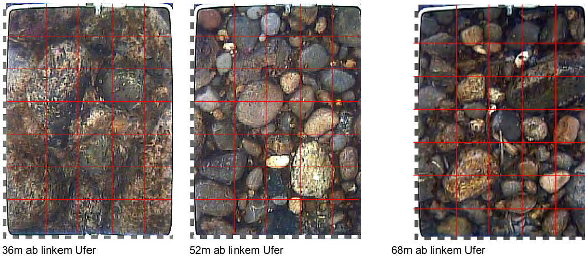
Bild 6.17 Unterwasserfotos in der Stauhaltung des Kraftwerks Reckingen (km 82.3). In der linken Gerinnenhälfte ist das grobkörnige Sohlenmaterial ersichtlich (Foto links), auf der rechten Gleithangseite ist die Sohle mit Glattgeschiebe überdeckt. Rasterweite 5cm.
