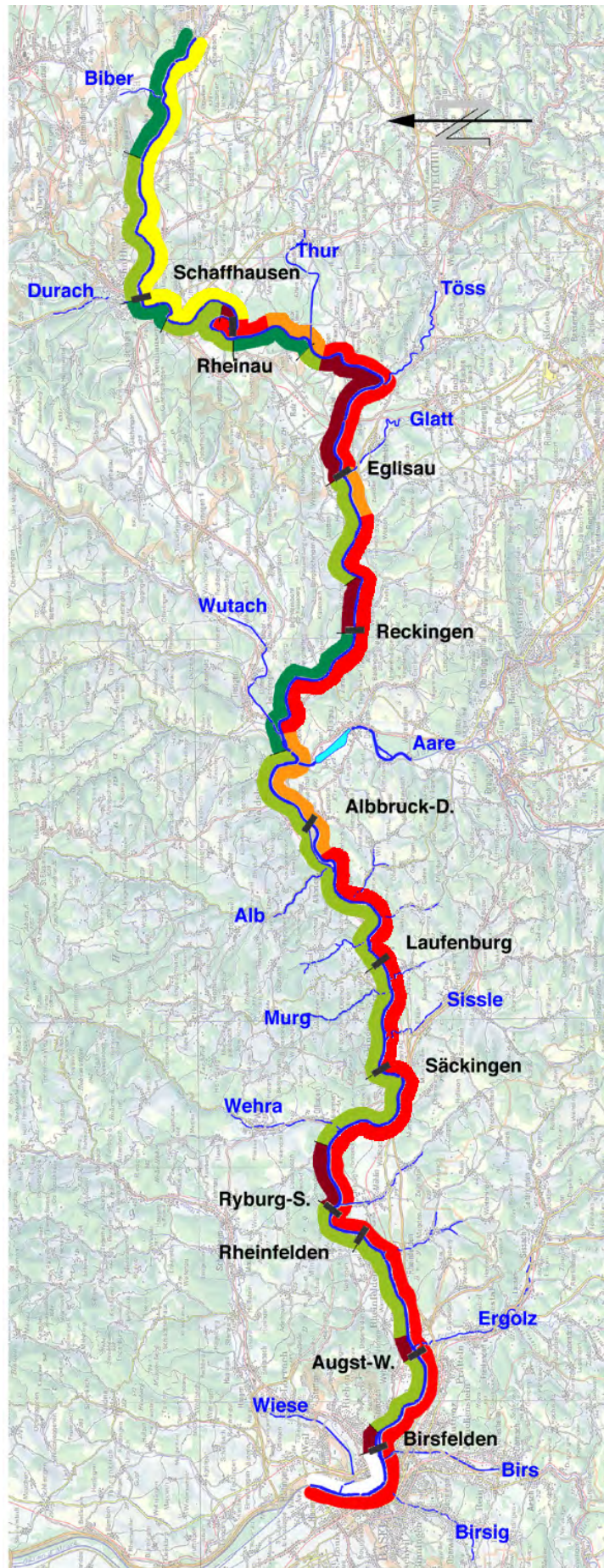
Bild 6.23 Aktueller Geschiebehaushalt des Hochrheins in der Situation. Rechts vom Rhein (in Fliessrichtung) ist die Geschiebetransportkapazität qualitativ dargestellt, links vom Rhein die Veränderung der Geschiebefracht gegenüber den Verhältnissen um 1900.
