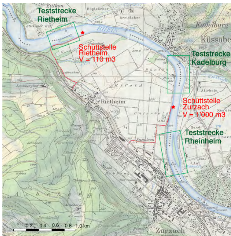
Bild 8.6 Lage und Zufahrtsstrecken zu den Schüttstellen Zurzach und Riethem sowie Lage der Teststrecken für die morphologischen und ökologischen Untersuchungen.
