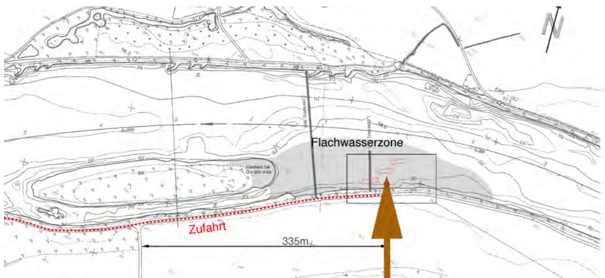
Bild 8.9 Lage der Schüttstelle Riethem im Bereich der bestehenden Flachwasserzone mit geringer Strömungsbeanspruchung. Massstab 1:5'000.
