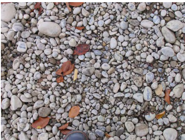
Bild 6.21 Geschiebeablagerungen im Unterwasser des Kraftwerks Ryburg-Schwörstadt (km 144.1) nach dem Hochwasser vom August 2005 ( Q_{max} = 3'464m^3/s ).
