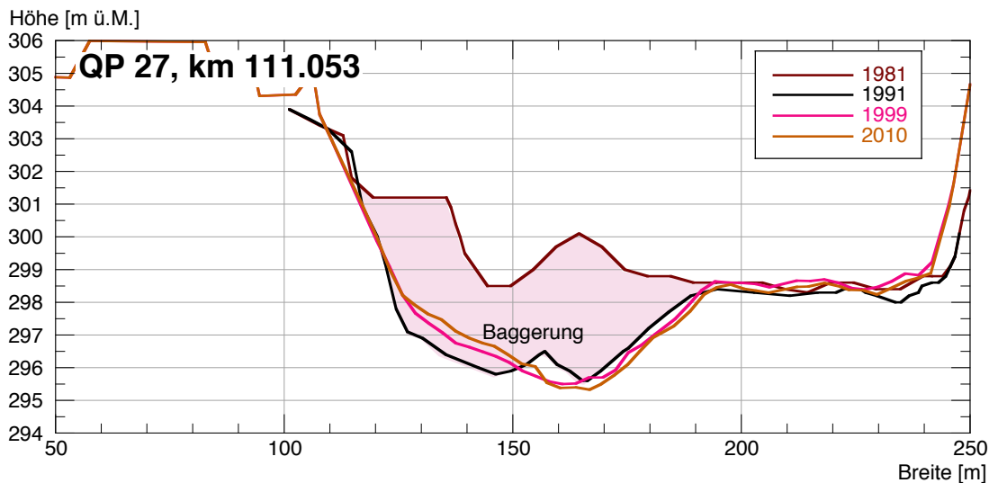
Bild 6.10 Querprofile 23, 25 und 27 in der Restwasserstrecke des Kraftwerks Albrück-Dogern mit Aufnahmen vor und nach der Sohlenbaggerung. Mit der Baggerung wurde die Sohle um gegen 6m abgetieft. Die Baggerlöcher wurden bis heute nur teilweise aufgefüllt. Die Profiänderungen am linken Ufer sind auf abgeschwemmte Feinsedimente während dem Hochwasser 1999 zurückzuführen.
