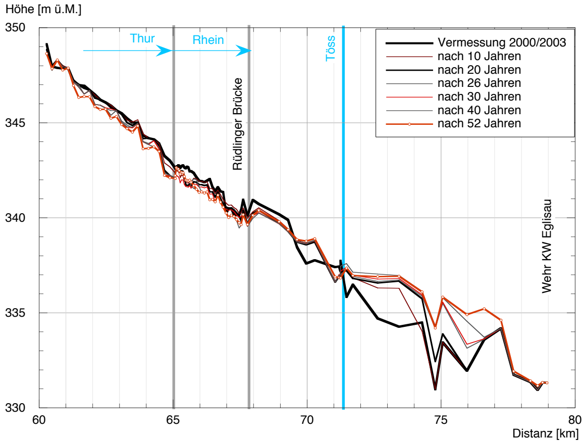
Bild 3.1 Längensprofil der mittleren Sohle im Mündungsabschnitt der Thur und der Stauhaltung Eglisau: Vermessene Sohle und berechnete Sohlenlage zu verschiedenen Zeitpunkten für den Fall mit Geschiebeeinträgen aus der Thur von 13'000 m 3 /Jahr und aus der Töss von 3'000 m 3 /Jahr.
