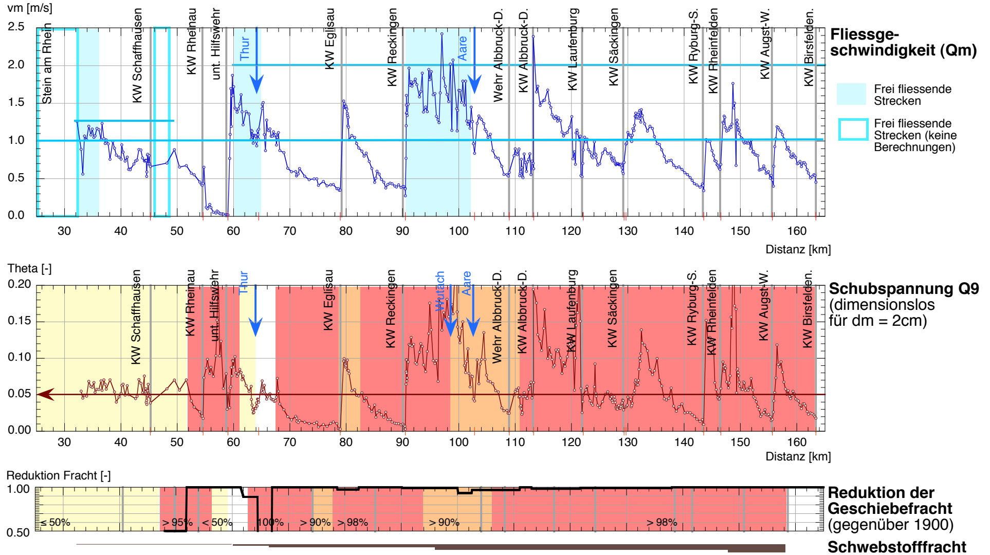
Bild 6.25 L\u00e4ngenprofile von berechneter mittlerer Flie遝geschwindigkeit bei Mittelwasserabfluss ( Q_m ) und dimensionsloser Schubspannung bei Q_9 ( \Theta ), Reduktion der urspr\u00fcnglichen Geschiebefracht (ohne Eintrag aus Ufererosionen) und qualitativer Beschreibung der Schwebstofffracht.
