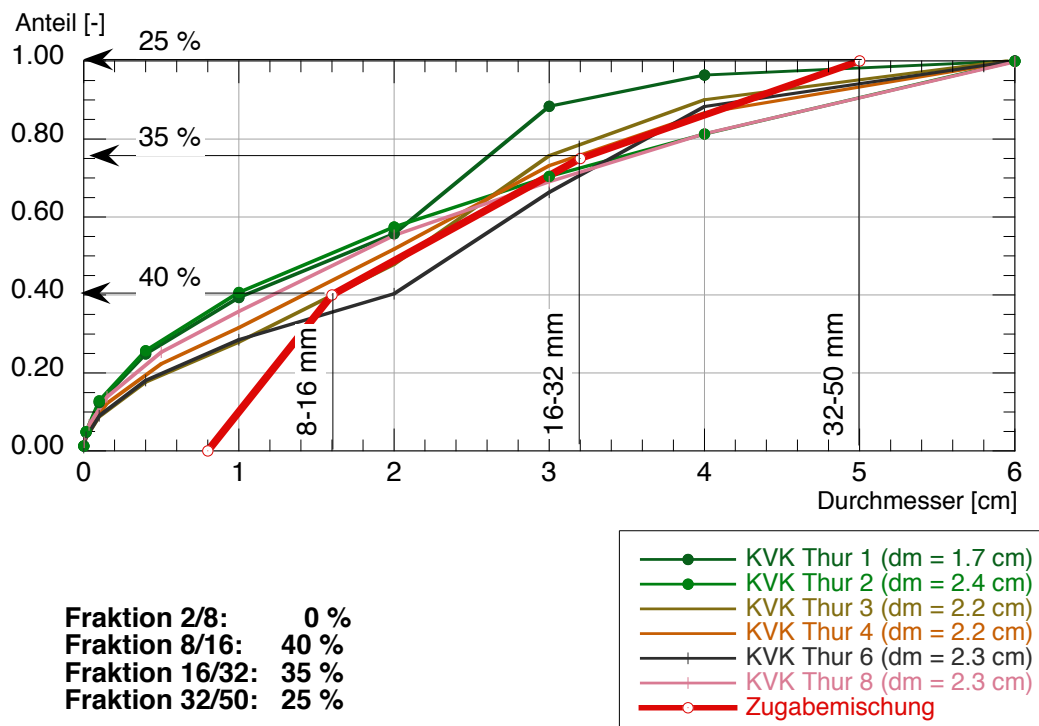
Bild 8.7 Kornverteilungskurven (KVK) von verschiedenen Proben des Thurgeschiebes sowie des verwendeten Schüttmaterials, das aus den vorhandenen Kiesfraktionen zusammengesetzt wurde.
