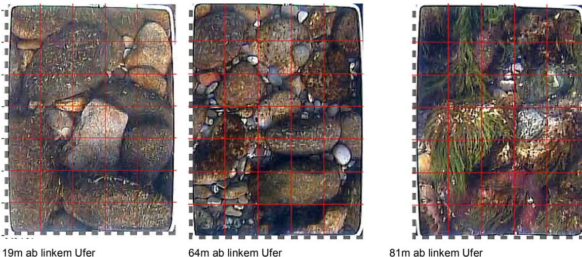
Bild 6.18 Unterwasserfotos in der frei fließenden Strecke bei Zurzach, oberhalb der Rheinheimer Insel (km 94.5). Im grobkörnigen Sohlenmaterial sind einzelne Geschiebekörner eingelagert. Rasterweite 5cm.
